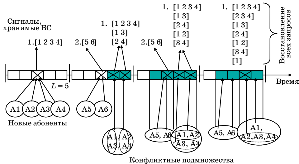
■ Рис. 4. Функционирование алгоритма Multi-FS-ALOHA/SIC (здесь к концу четвертого кадра КП с четырьмя запросами обслуживается за счет использования SIC)
