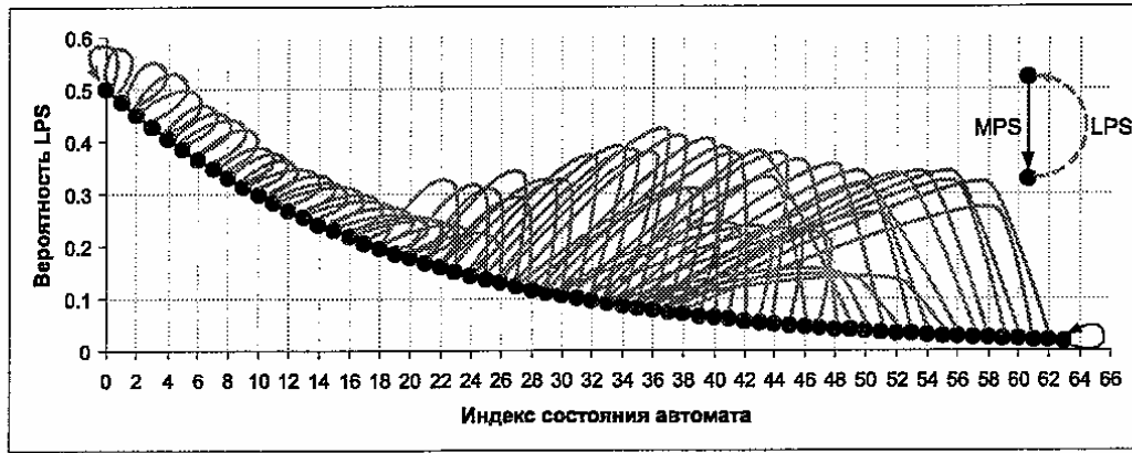
Рис.1 Оценка вероятности в стандарте H.264/AVC
